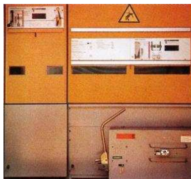
Cellules de comptage et de protection
